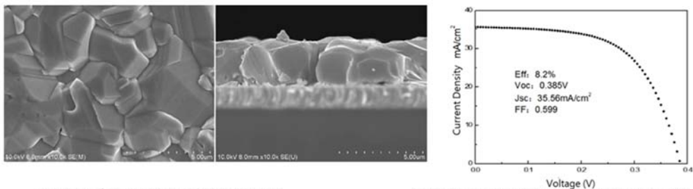
(a) CZTSe 薄膜之 SEM 表面形貌及橫截面圖 (b) 3 階段硒化法之 CZTSe 太陽能電池的 I-V 曲線 目前全世界高效率之 CZTSe(S) 太陽能電池製作方法的比較表
